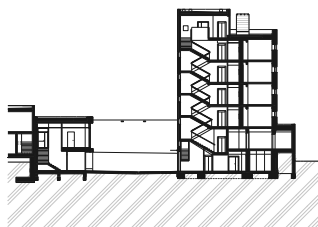
Řez
