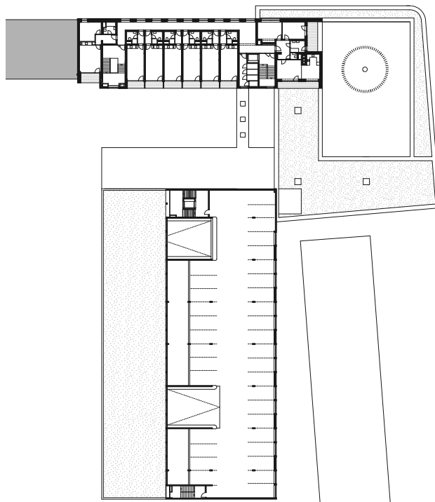
Půdorys 2. NP
