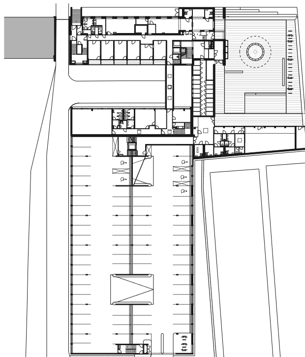
Půdorys 1. NP
