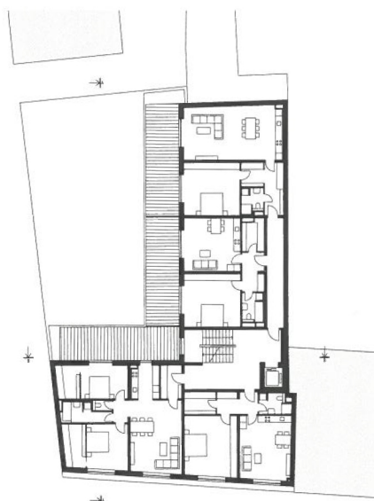
Půdorys 2. NP
