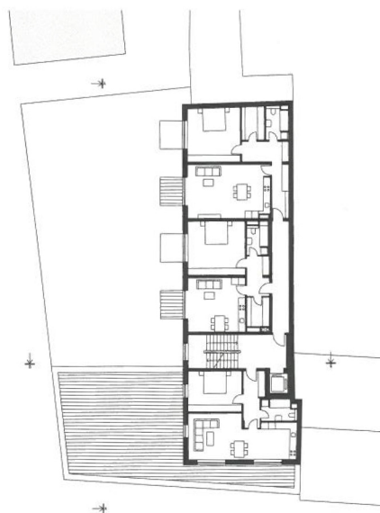
Půdorys 4. NP
