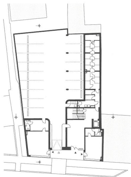
Půdorys 1. NP
