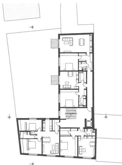
Půdorys 3. NP
