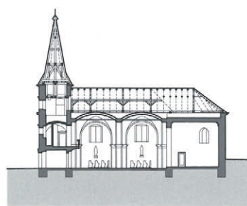
řez section
